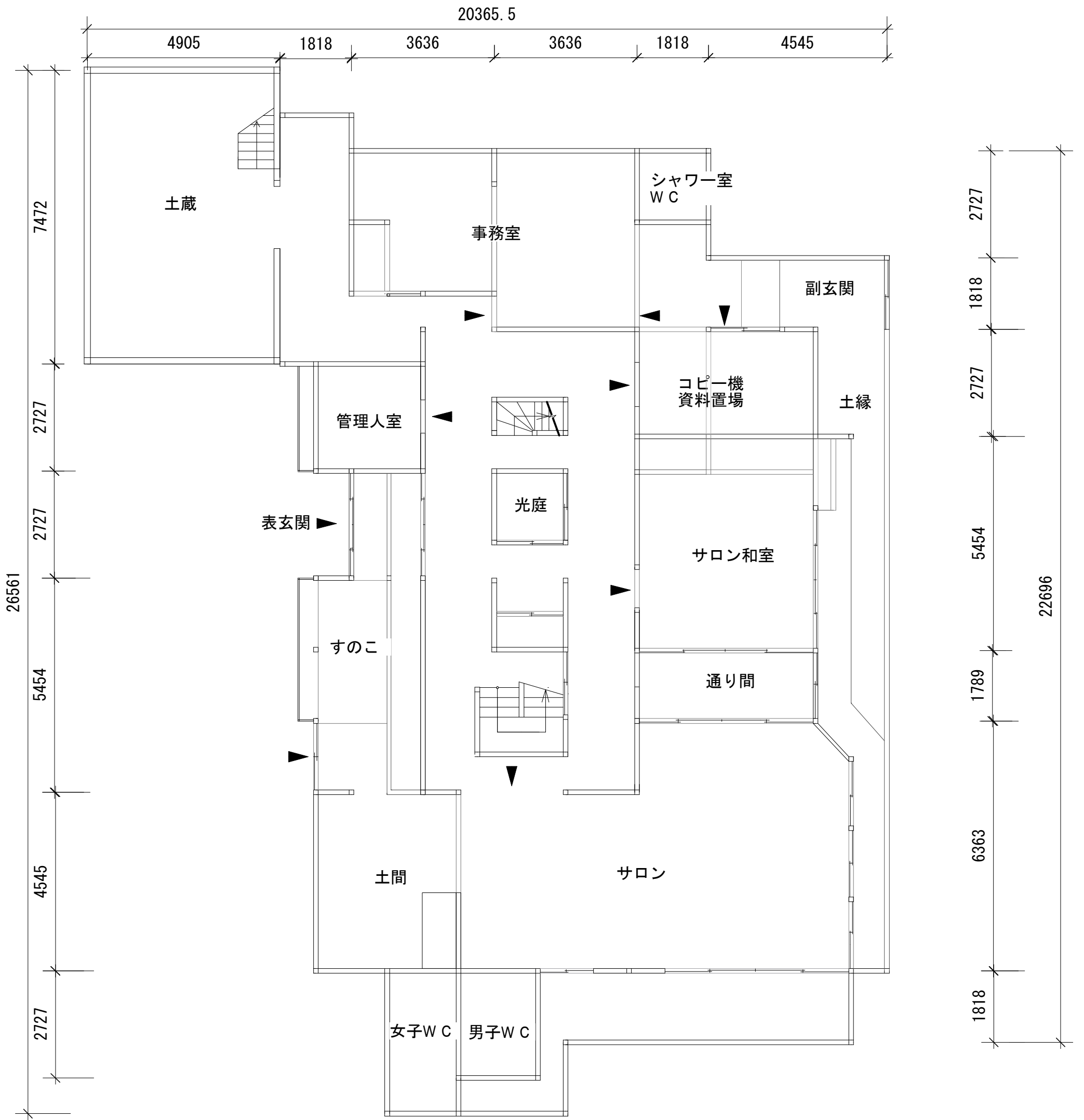
1F平面図 S1:100
