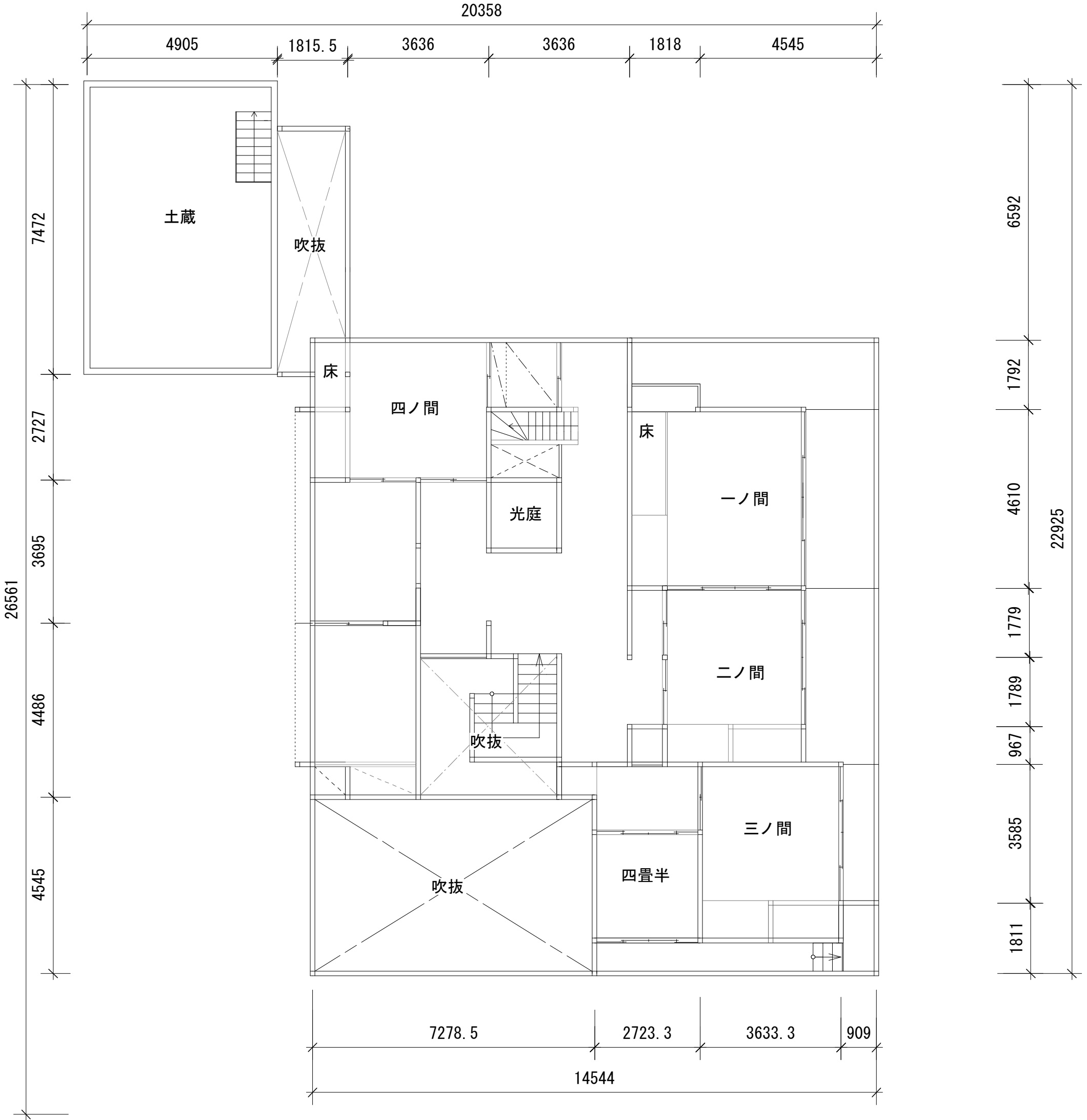
2F平面図 S1:100
