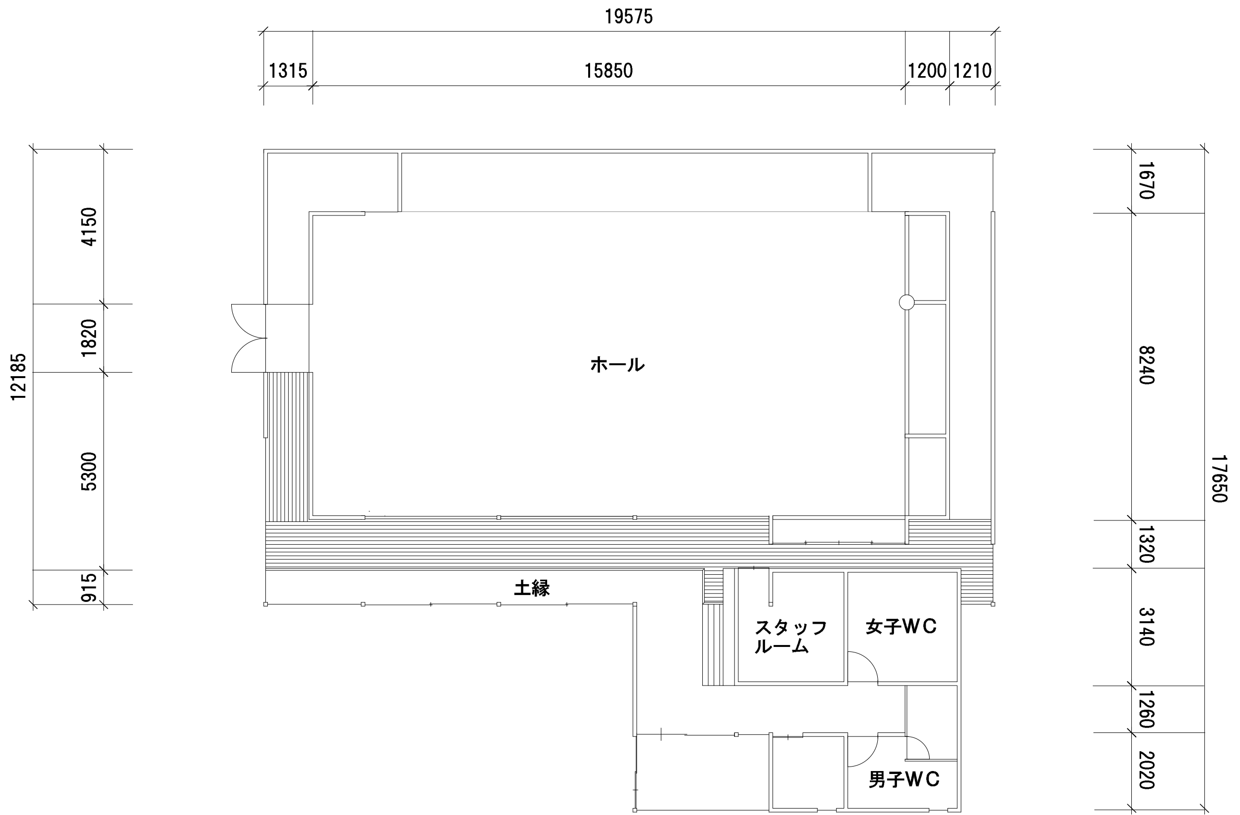
交流ホール平面図 1:100
