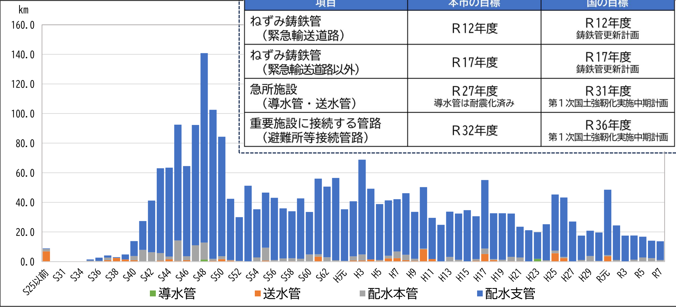
水道管路の年度別布設延長
