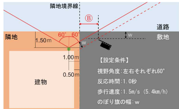
図2 隣地からの距離
