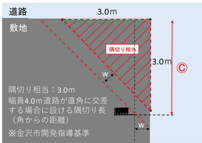
図3 道路交差点角地の隅切り相当範囲
