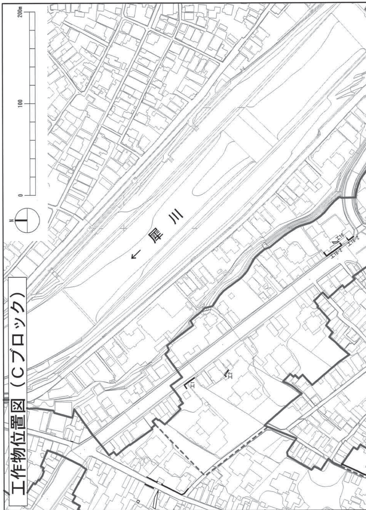
別図第3 - 4 伝統的建造物（工作物）に係る図面（Cブロック）
