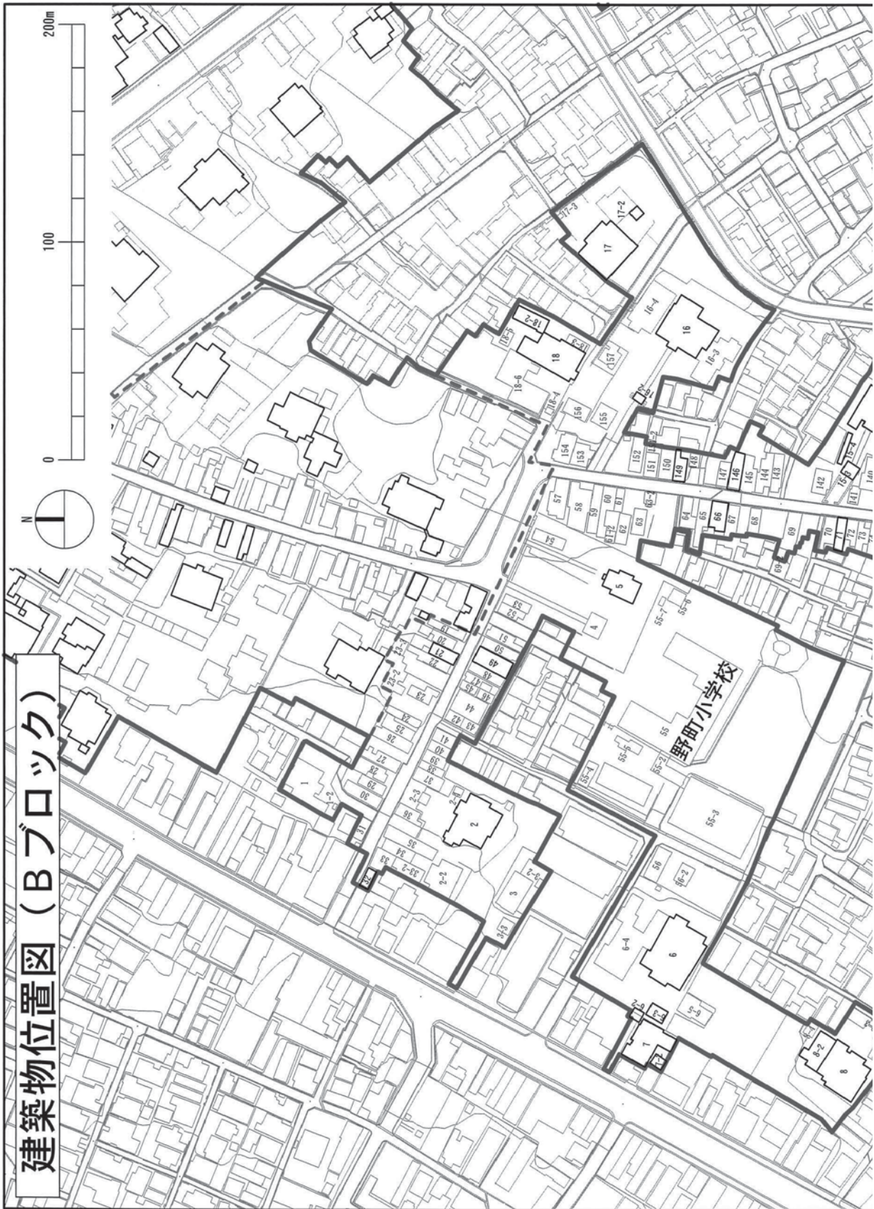
別図第2 - 3 伝統的建造物（建築物）に係る図面（Bブロック）
