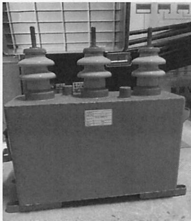
廃棄物 (3-009) 外観
