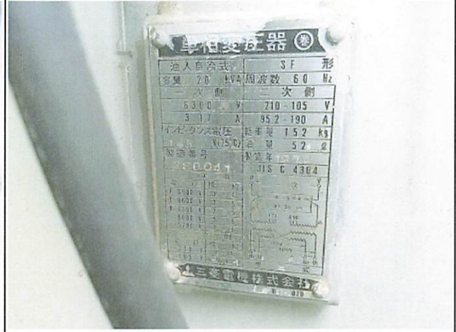
変圧器(5-001) 銘板写真
