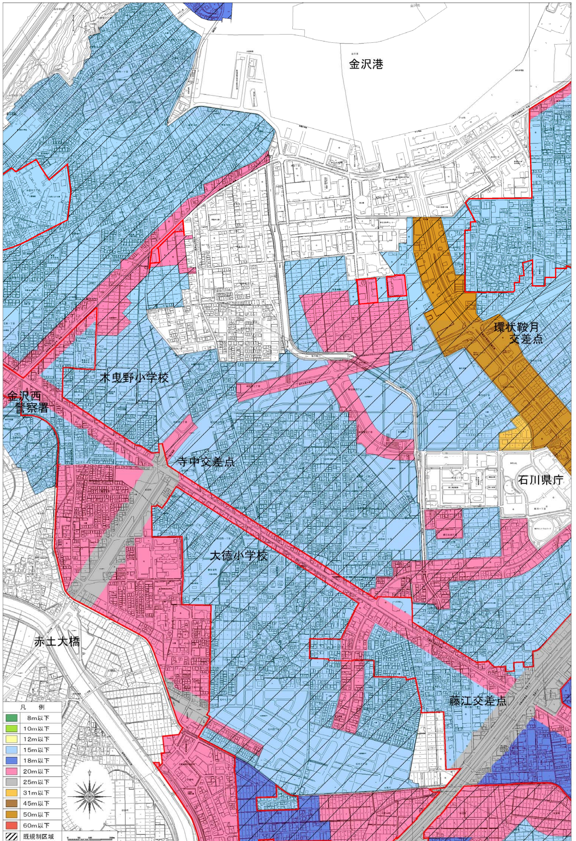
高さ制限案図(大徳地区)
