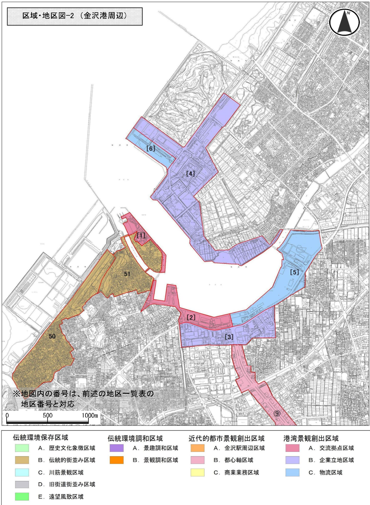
【景観形成区域詳細図2】
