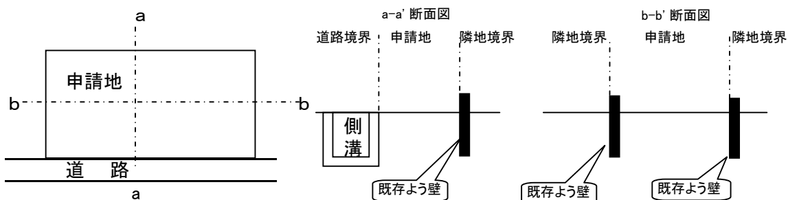
(記載例) 境界簡易断面図
