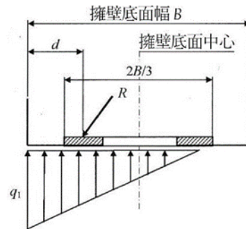
(b) 荷重の合力 R の作用位置が底版中央の底版幅 1/3 から 2/3 の範囲にある場合（三角形分布）
