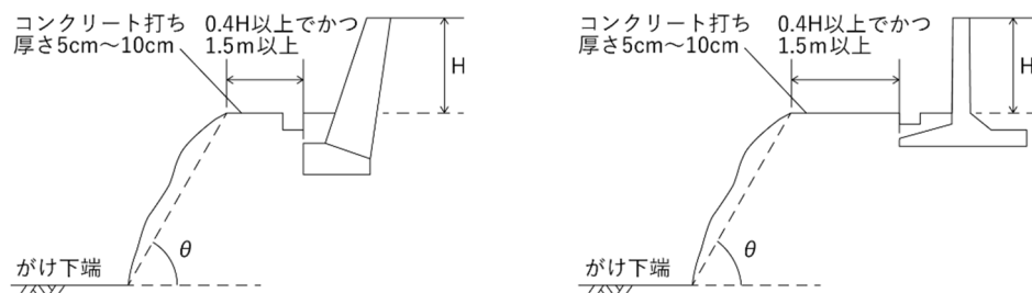
図2. 3-1 斜面の擁壁の構造
