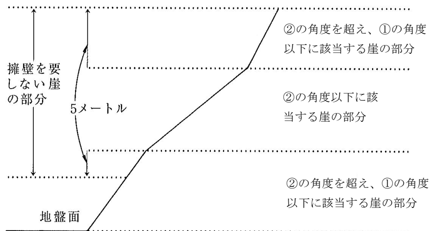
図 2.1-1 擁壁を要しない崖又は崖の部分
