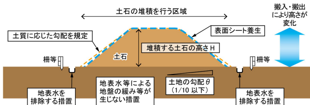
図 7.2-1 堆積した土砂の崩壊やそれに伴う流出を防止する措置の概念図
