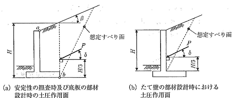
図 3.3-2 土圧の作用位置（片持ち梁式）
