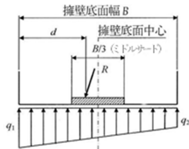
(a) 荷重の合力 R の作用位置が底版中央の底版幅 1/3 の中にある場合（台形分布）
