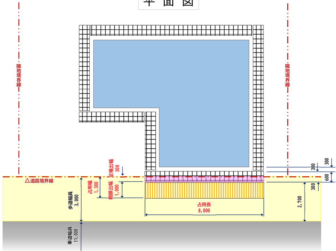
平面図
