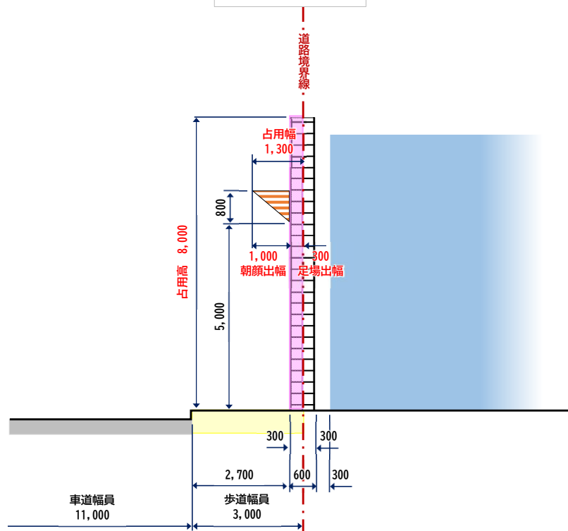
断面図
