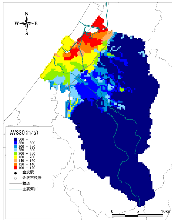
図 2-4-3 AVS30 分布
